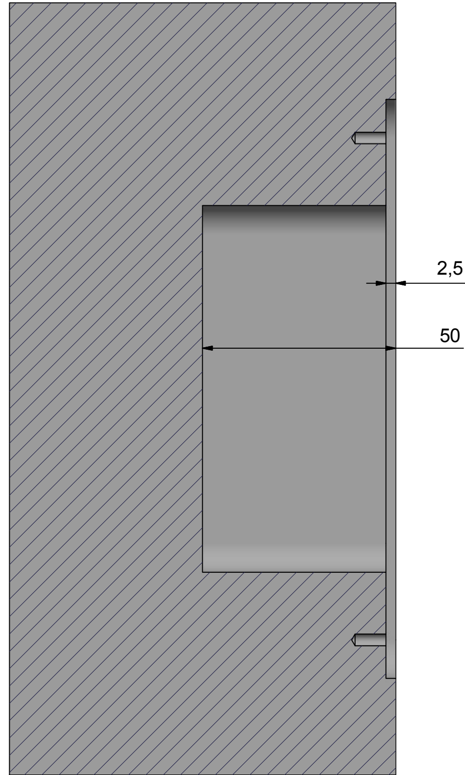
A-A (1:1)
